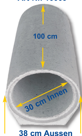
Beton-Falzrohr: Art-Nr. 10009
