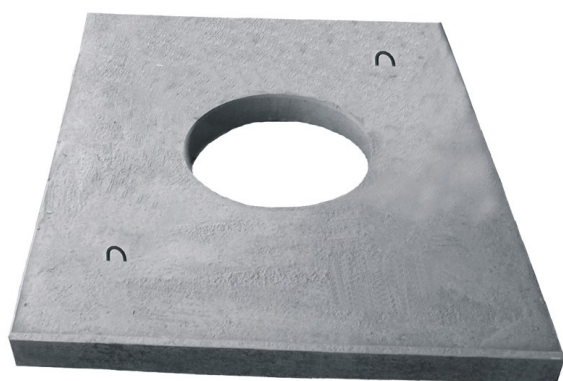
Kanalabdeckplatte mit zentrischer Einstiegs Luke und 2 Transportösen
