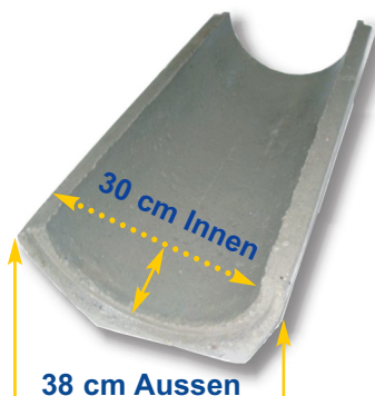
Beton-Halbschale: Art-Nr. 10360
