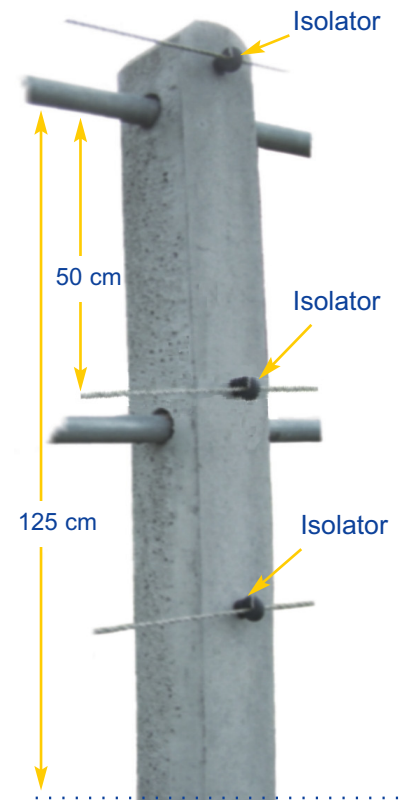
Pferdekoppelpfahl
