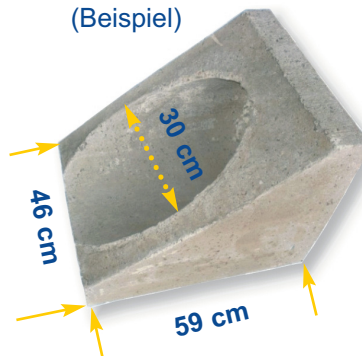
Böschungs-Ein/Auslauf: Art-Nr. 10150 (Beispiel)
