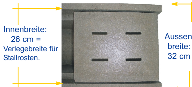
Stallroste mit Schlitz auf U-Kanal
